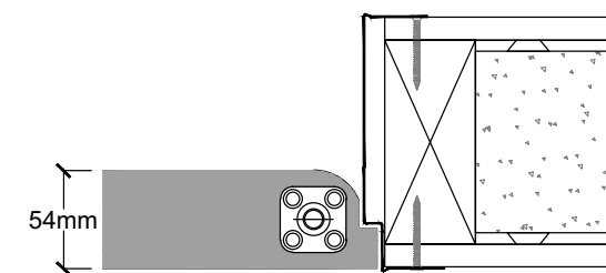
Dot & dab
