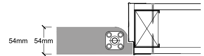
Metal stud partitioning
